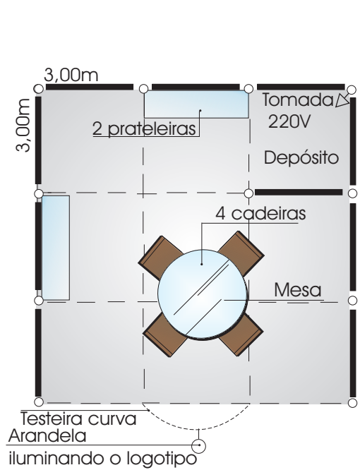
PLANTA BAIXA
